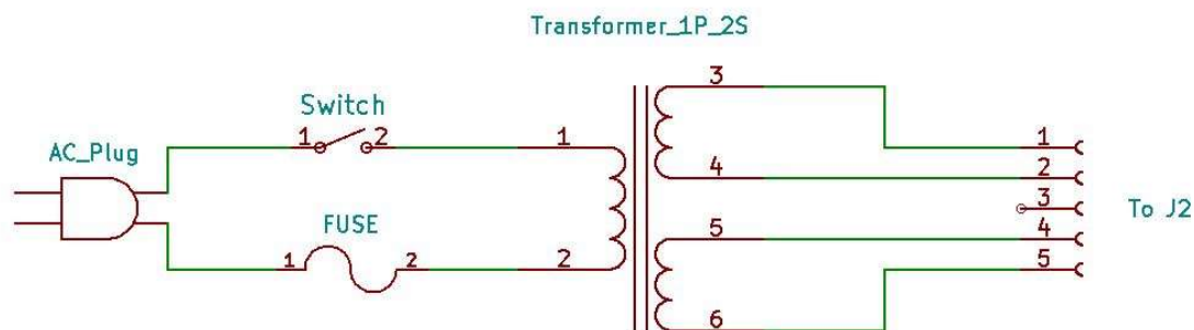
図1. 電源配線
